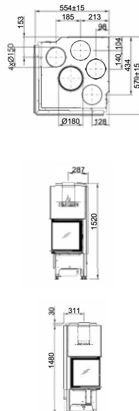
Linear Corner 46x46x57 (P. 38) Mini 2LRh-57-4S
