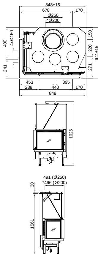
Linear Corner 46x46x51 (P. 38) Mini 2LRh-51-4S
