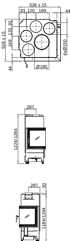
Swing Corner 46x46x51 (P. 38) Mini 2L/2R-4S
