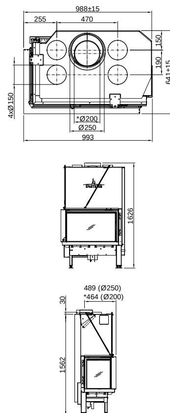
Linear Corner 46x46x57 (P. 38) Mini 2LRh-57-4S
