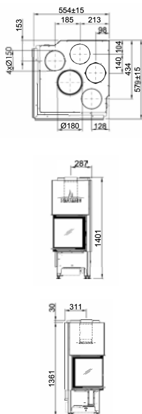
Linear Corner 46x46x51 (P. 38) Mini 2LRh-51-4S
