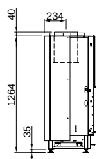
Linear Tunnel 60x51 (P. 62) Mini S-FDh-4S
